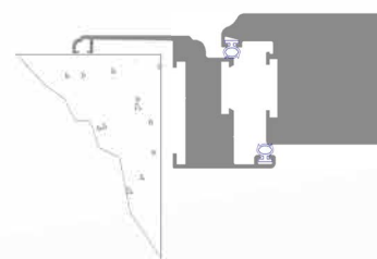
DETTAGLIO GEOMETRICO
